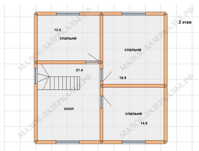
План 2 этажа
